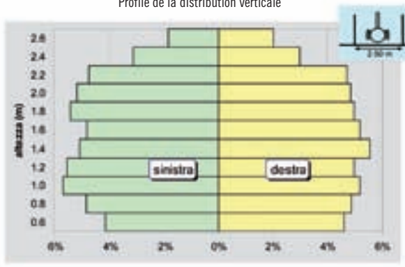
Velocità dell'aria rilevata a 0.50 m dall'uscita Air speed measured 0.50 m from outlet Luftgeschwindigkeit gemessen 0.50 m von Ausgang Vitesse du vent mesurée à 0.50 m de la sortie
