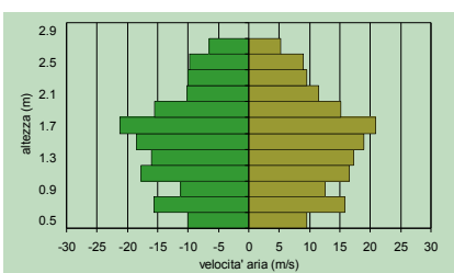
I - 1890 giri/min
