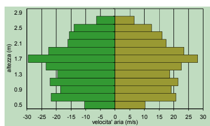
II - 2700 giri/min
